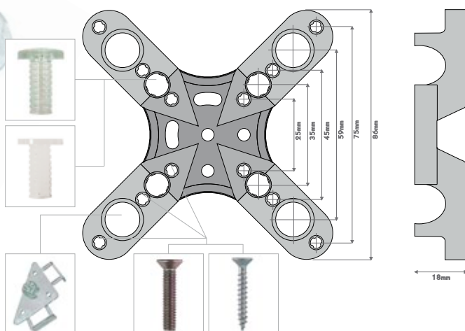
fissaggio di pannelli con il distanziale zigrinato fixxo. panelbefestigung mit fixxo klicksystem. panel mounting with fixxo click-in.
